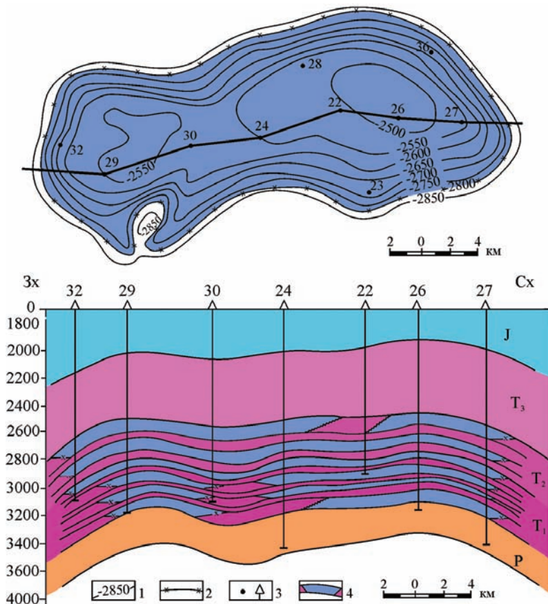
Рис. 6. Мурманське газове родовище. Структурна карта покрівлі I продуктивного горизонту в середньотриасових відкладах та геологічний розріз (склав М.І. Павлюк з використанням матеріалів А.В. Борисова, Ф.А. Грузер, В.М. Мартіросяна, Т.Н. Танигіної).
