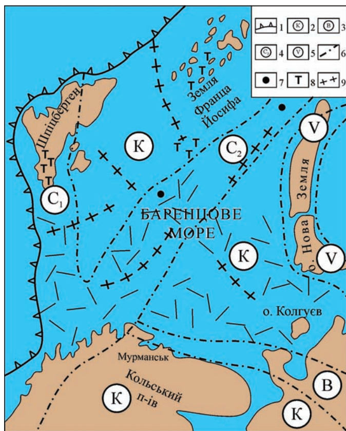
Рис. 2. Схема районування фундаменту Баренцове-морського шельфу (склав М. І. Павлюк за використанням матеріалів ВНДІ Океанології, ВО Союзморгео, ВО Північморгео, ВО Арктикморнафтогазрозвідка).
