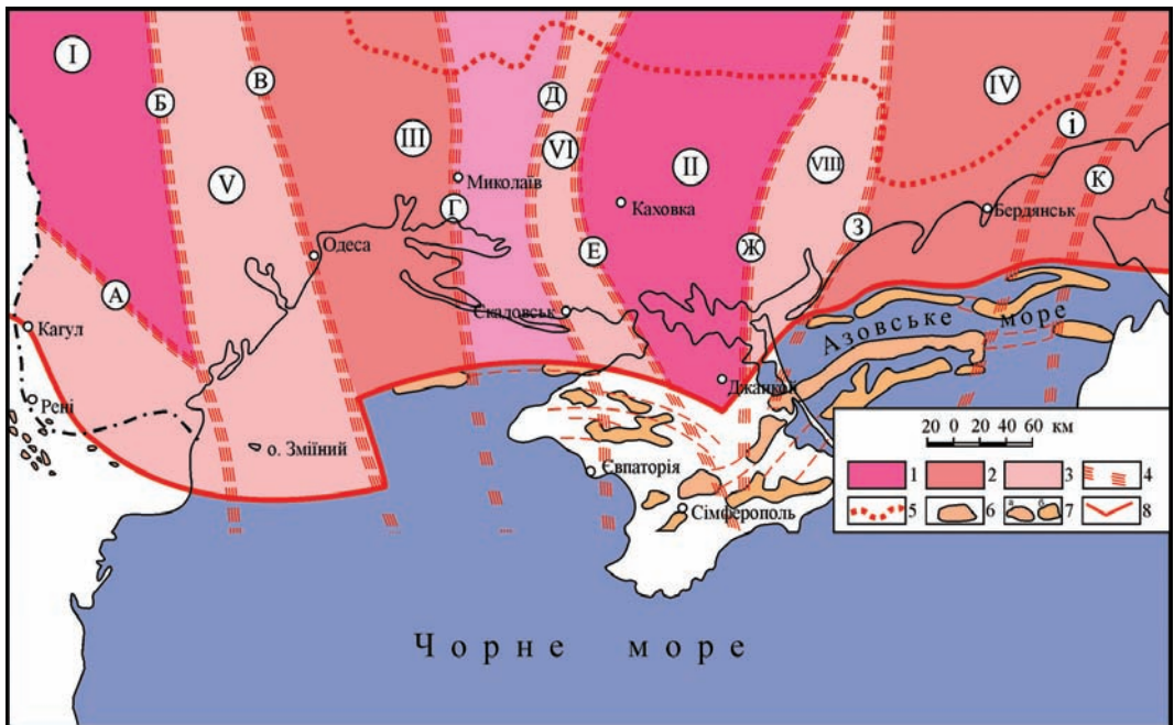
Рис. 4. Схема будови фундаменту південного краю Східноєвропейської платформи (склав М.І. Павлюк з використанням матеріалів О.Т. Богайця, І.А. Гаркаленка, Г.І. Каляєва, М.В. Муратова, Л.Г. Плахотного, В.А. Рябенка, В.І. Старостенка, К.Г. Тяпкіна, А.В. Чекунова).
