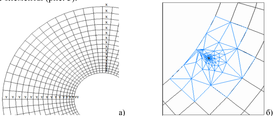
Рис. 3 – Фрагмент конечно-элементной модели диска (а) и стартовая трещина (б).
