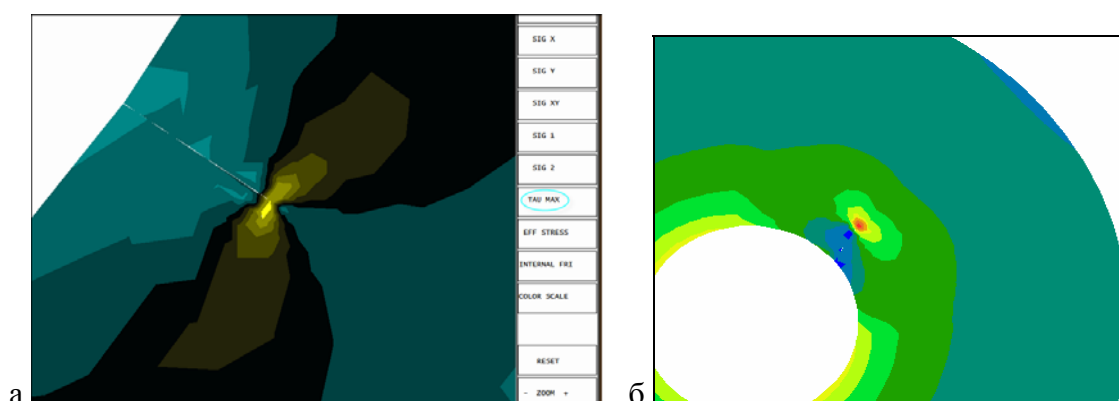
Рис. 4 – Распределение в образце максимальных касательных напряжений \tau_{\max} при начальном нормальном (а) и наклонном расположении трещины (б).
