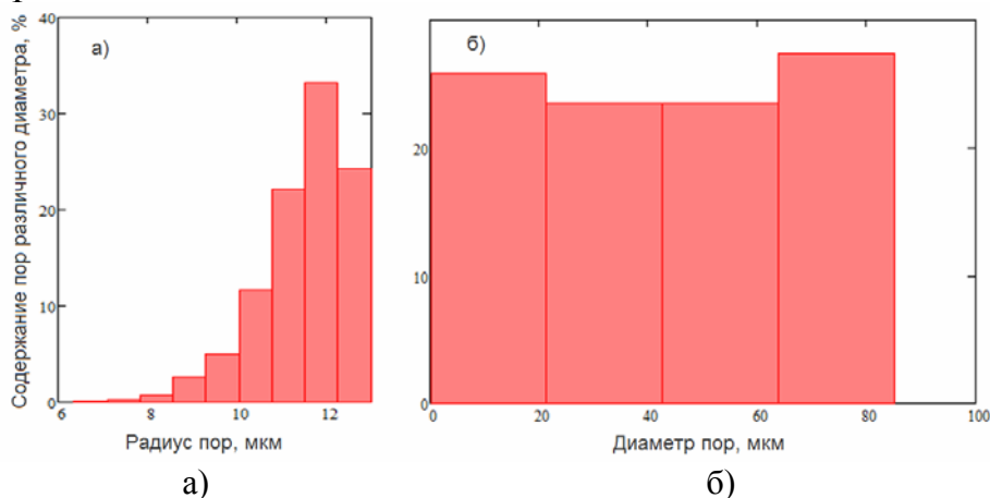
Рис. 2 – Гистограммы распределения пор мелкозернистого (а) и крупнозернистого (б) песчаников.
