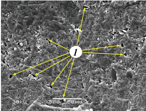
Рис. 6. Поры раскрытых газово-жидких включений (1) в кальците грязевого вулкана Пыккле Мичи
