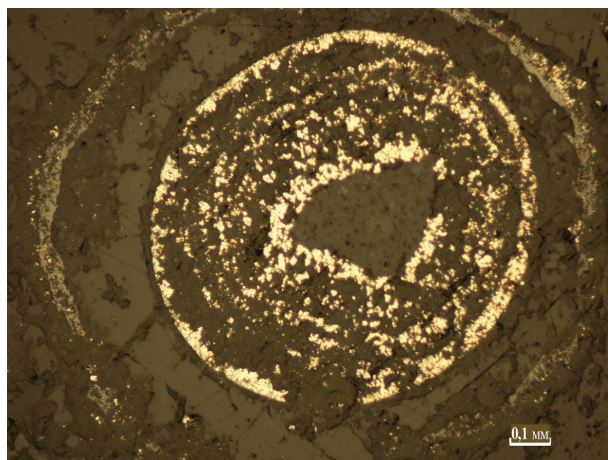
Рис. 2. Пирит из твердых выбросов сопочной брекчии грязевого вулкана Пыккле Мари
