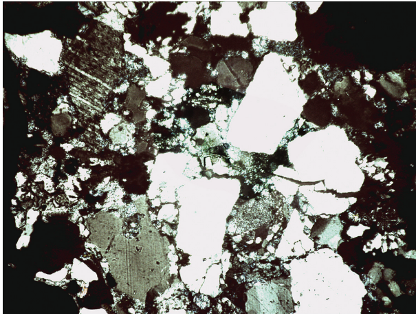
Рис. 7. Песчаник из твердых выбросов сопочной брекчии грязевого вулкана Пыккле Мичи. Николи+
