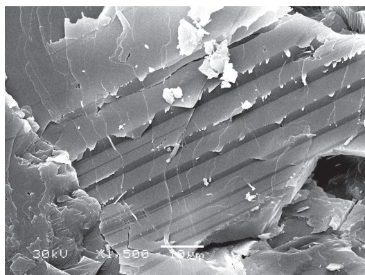
Рис. 4. Массивный жильный кальцит из твердых выбросов грязевого вулкана Пыккеле Мичи
