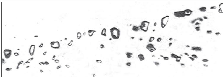
Рис. 8. Типичное расположение групп вторичных флюидных включений в породообразующем кварце. Увеличение 120
