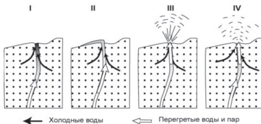
Рис. 2. Механизм действия гейзера
