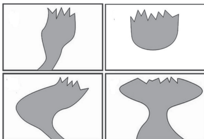
Рис. 3. Принципиальная схема "плюма" [1]
