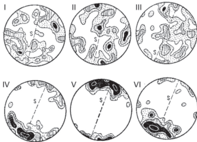
Рис. 6. a — Диаграммы ориентировки оптических осей кварцевых зерен в неизменных породах: I— аляскитовый гранит, II— гранодиорит, III— кварцевый микродиорит, и в бластомилонитах IV—VI. По [10]. б — Ритмическое отложение минералов в рудной жиле. По [8]. Слева — зарисовки жилы. 1, 3 — кальцит, 2 — настуран, 4 — кальцит с коффинитом, арсенидами и сульфидами. Справа — микрофото зоны корки настурана. Увеличение 200
