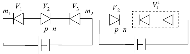
Рис. 4. Упрощенная эквивалентная схема трехбарьерной структуры, приведенной к двухбарьерной
