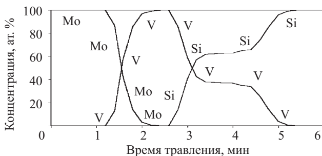
Рис. 4. Профиль распределения элементов многослойной структуры Mo/V/Si после температурной обработки при 625°С в течение 30 мин
