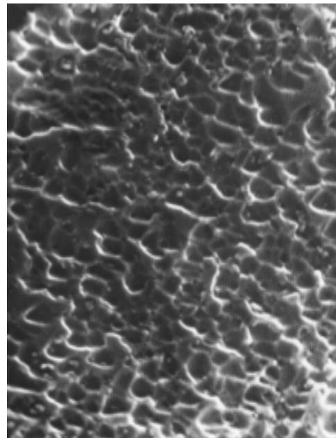
Рис. 3. Периодическая островковая структура, состоящая из областей наноструктурированного бездефектного кремния на поверхности пластины кремния КЭФ-4,5 (111)
