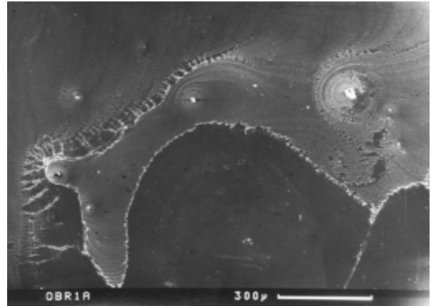
Рис. 2. Дефекты слоистой неоднородности на поверхности кремниевой пластины КЭФ-4,5 (111), полученные после травления ИТ Сиртля в течение 2 мин
