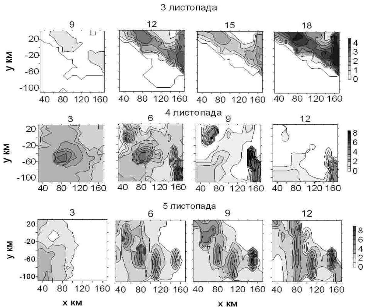
Рис. 4. Змодельовані тригодинні суми опадів синоптичного процесу 3-5 листопада 1998 р. (Цифри біля вершин рисунків означають кінцевий термін змодельованої суми. Цифри біля шкал – суми опадів, мм)
