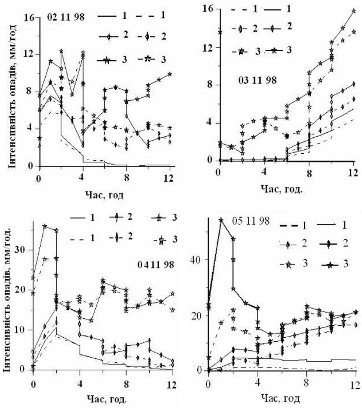
Рис. 6. Змодельована еволюція інтенсивності опадів 2-5.11.1998 р.: 1. Інтенсивність опадів у точці (x, y) = (100, -30 \text{ км}) . 2. Макс. інтенсивність опадів на малій площі (100 < x < 150 \text{ км}, -30 < y < 20 \text{ км}) . 3. Макс. інтенсивність опадів для всієї розрахункової площі (-170 < x < 300 \text{ км}, -250 < y < 220 \text{ км}) . (Суцільні лінії – розрахунки без коагуляції, несучільні – з коагуляцією)
