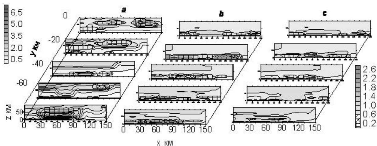
Рис. 8. Просторовий розподіл водності, г/кг (шкала – праворуч) та концентрації кристалів, 1000/г (шкала – ліворуч); t = 3 год. 5 листопада 1998 р. a - A = 2 м/с, B = 10 м/с, c = 0 ; b – як a , при A = 0,75 м/с; c – як b , при c = 1
