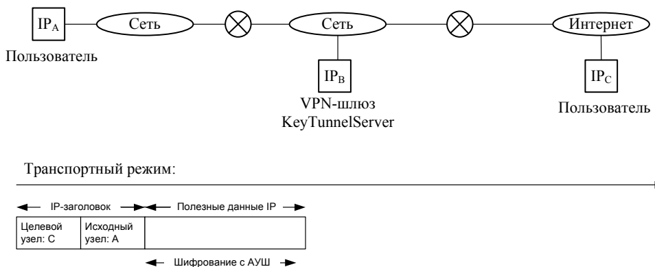
Рис. 10. Транспортный режим модифицированного протокола IPsec
