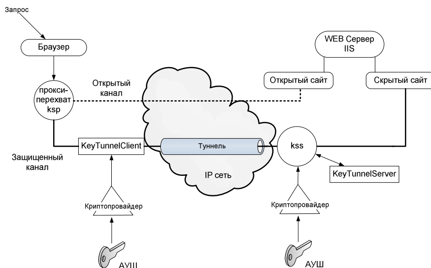
Рис. 15. Организация защищенного канала передачи данных со скрытым Web-узлом
