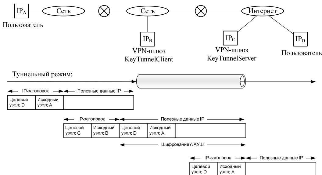
Рис. 11. Туннельний режим модифікованого протокола IPsec
