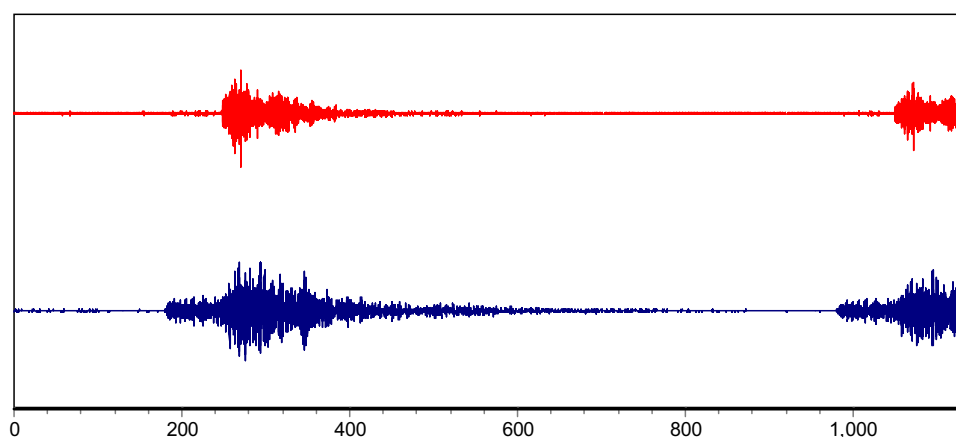
Рис. 10. Отклики диагностируемого участка на удар: до и после компенсатора
