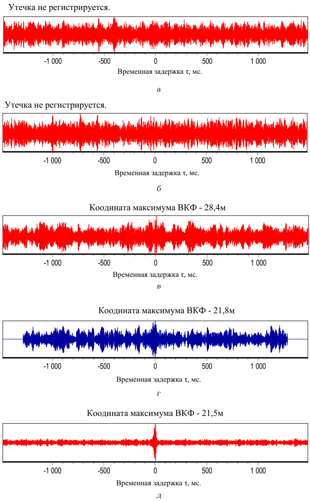
Рис. 8. Виды ВКФ вибросигналов, полученные при различных положениях вибродатчиков в теплокамерах: а-г – промежуточные результаты, д – конечный результат
