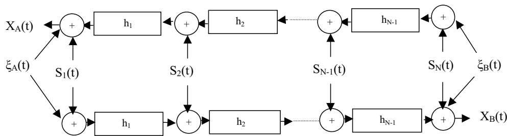
Рис. 3. Модель диагностируемого участка теплосетей с учетом частотной зависимости параметров канала распространения вибросигналов
