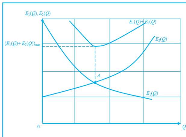
Рис. 3. Типові графіки залежностей економічностей установок осушення попутного газу E_1 і сепараційної установки E_2 як підсистем НГВП від продуктивності Q – приклад формування синергічного ефекту при горизонтальній інтеграції двох підсистем
