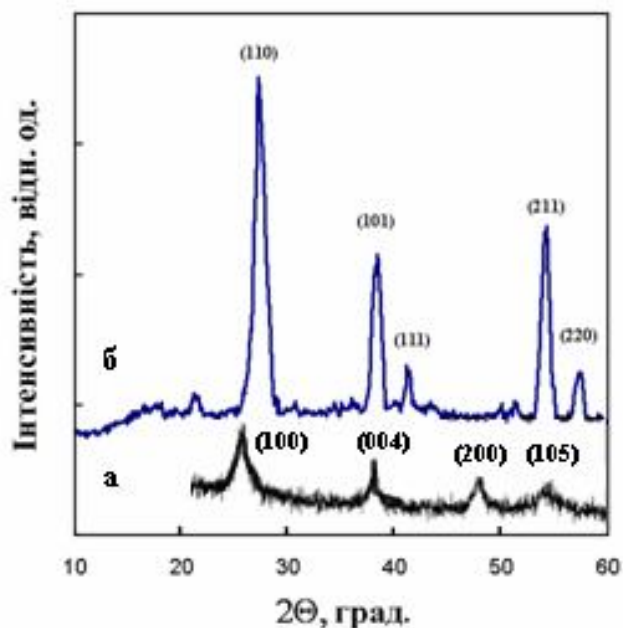
Рис. 4. Дифрактограма матеріалу з нанорозмірних частинок діоксиду титану: а – зразків, висушених при температурі 400 К; б – після високотемпературного відпалювання.
