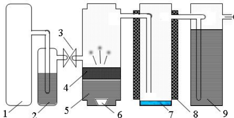
Рис. 1. Схема установки для вивчення гідролізу тетрахлориду титану на поверхні аерозолі: 1 - джерело газу-носія (повітря, аргон), 2 – осушувач, 3 – ротаметр, 4 – розчин тетрахлориду титану в гідрофобному розчиннику, 5 – вода, 6 – УЗ диспергатор, 7 – вода або водний розчин аміаку, 8 – нагрівач, 9 – уловлюючий розчин.
