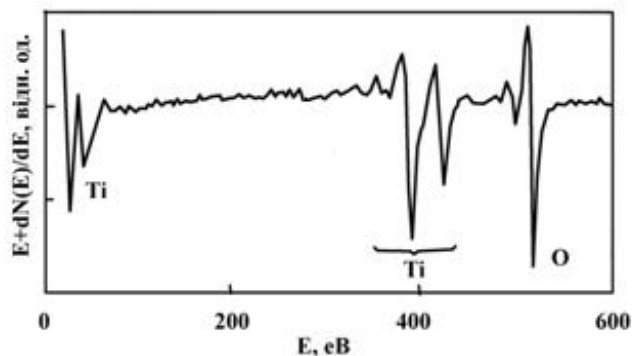
Рис. 6. Оже-спектри поверхні наночастинок діоксиду титану після відпалювання при температурі 1000 К.
