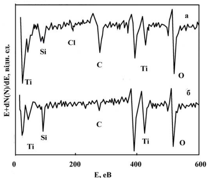
Рис. 5. Диференціальні Оже-спектри наночастинок діоксиду титану, осаджених на поверхню пластини монокристалічного кремнію: а – поверхні частинок; б – після травлення поверхні іонами Ag на глибині 200 нм.
