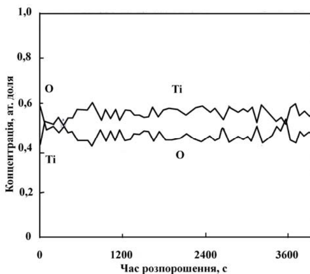
Рис.7. Відхилення стехіометрії \text{TiO}_2 від часу травлення плівки.
