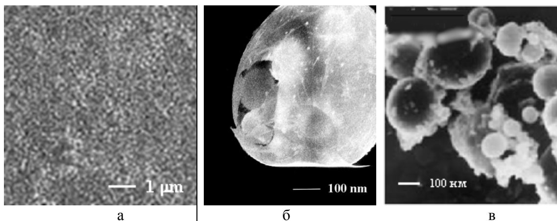
Рис. 2. Порожнинні сферичні частинки діоксиду титану (РЕМ зображення).
