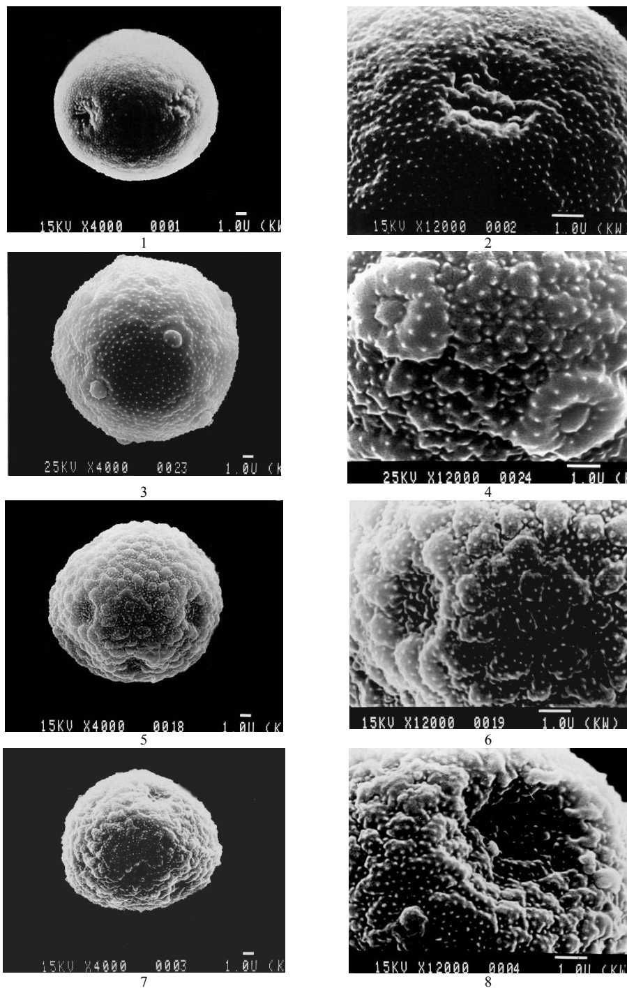
Пилок представників роду Plantago L. (СЕМ): 1, 2 — P. cornuti Gouan; 3, 4 — P. lanceolata L.; 5, 6 — P. major L.; 7, 8 — P. maxima Juss. & Jacq.; 9, 10 — P. media L.; 11, 12 — P. neumannii Opiz; 13, 14 — P. salsa Pall.; 15, 16 — P. tenuiflora Waldst. & Kit.
