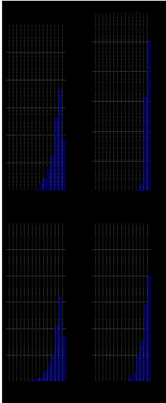
Рис. 4. Вертикальний розподіл фітомаси бобових за ступенями пасквального градієнта (а — ПД0; б — ПД1; в — ПД2; г — ПД3; д — ПД4) Fig. 4. Vertical distribution of legumes phytomass on the stages (a — PD0; б — PD1; в — PD2; г — PD3; д — PD4) of grazing gradient
