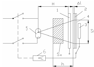
Рис.1. Принцип работы прибора для автоматической определения экспозиции при рентгенологических исследованиях
