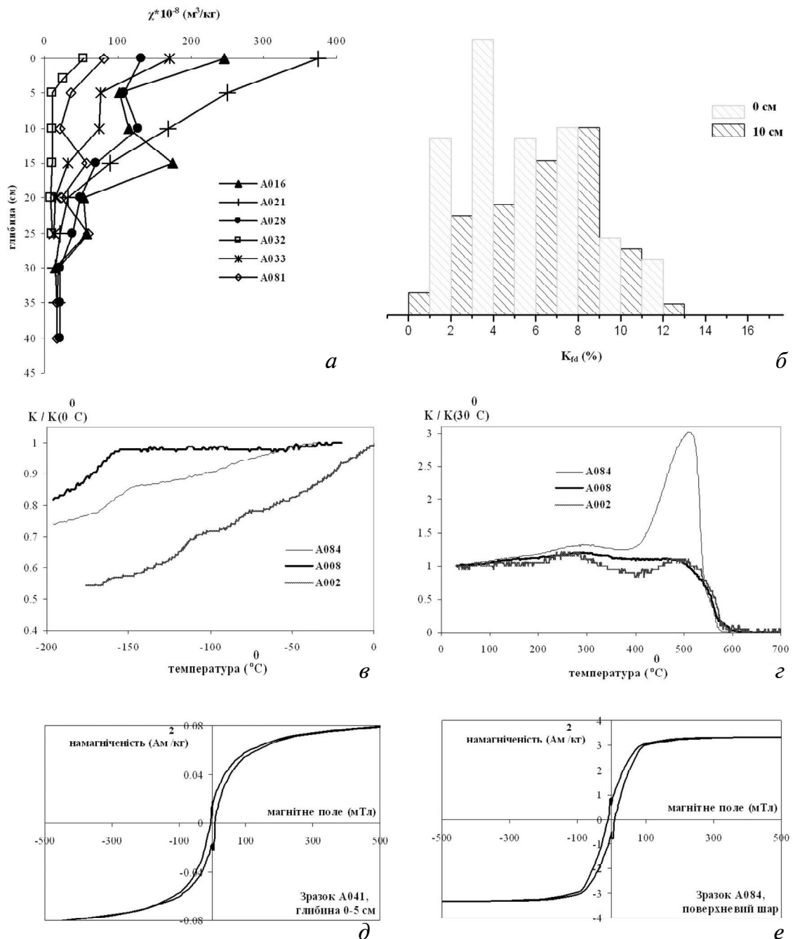
Рис. 2. Петромагнітні властивості ґрунтів Північної Астурії (пункти А008, А016, А021, А081, А084 розташовані в зонах впливу промислових підприємств, пункти А002, А032, А033, А041 – фонові)
