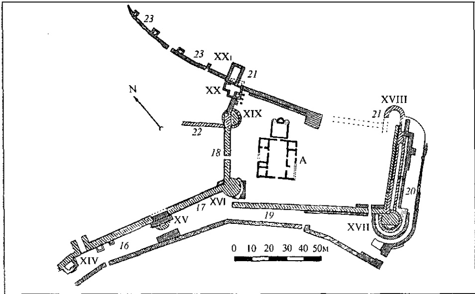
Рис. 2. План Херсонської «цитаделі»: XIV—XX — вежі; 16—23 — куртини; А — «фемний будинок»
