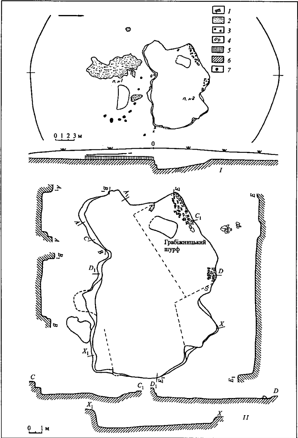
Рис. 3. Іванівка, курган № 7: I — план та профіль кургану; II — план та розрізи поховання № 2; 1 — дерево перекриття; 2 — шар вугілля від спаленої дерев'яної конструкції; 3 — скопичення керміки; 4 — каміння; 5 — поховальна почва; 6 — материк; 7 — стовпові ями
