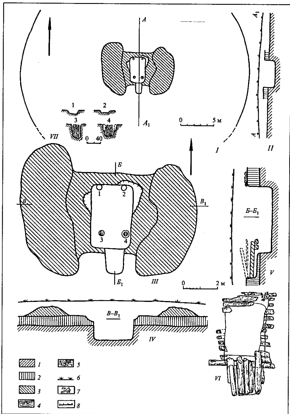
Рис. 1. Іванівка, курган № 1: I, II — план та профіль кургану; III—V — план та розрізи могили; VI — залишки дерев'яного перекриття могили; VII — стовпові ями (1—4). Умовні позначення: 1 — материк; 2 — поховальна почва; 3 — материковий викид; 4 — дерево перекриття; 5 — обпалене дерево; 6 — орний шар; 7 — людські кістки; 8 — обрис грабіжницьких ходів
