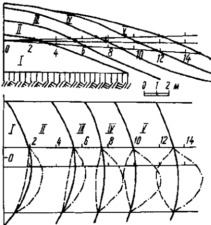
Рис. 1. Залежність реконструкції контурів насипів від відхилення горизонталі (умовна модель).
