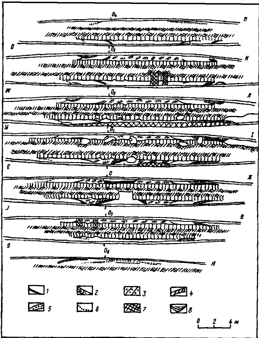
Рис. 7. Профілі бровок к. 6 біля с. Високе.
