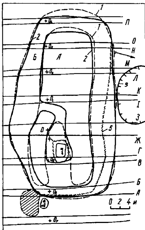
Рис. 6. Загальний план к. 6 біля с. Високе Умовні позначення: А — внутрішня споруда; Б — зовнішня споруда; 1 — контури першого, звітного варіанта реконструкції; 2 — другий варіант реконструкції; 3 — материкова виборка; 4 — внутрішня межа викиду з основного поховання; 5 — контур чорноземної межі зовнішньої споруди з півночі.
