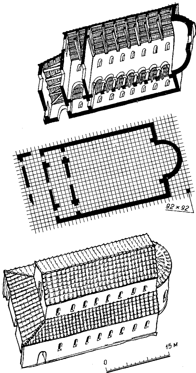
Рис. 4. Реконструкція «Базиліки 1935 р.». Аксиометричний переріз, план та аксонометрія.
