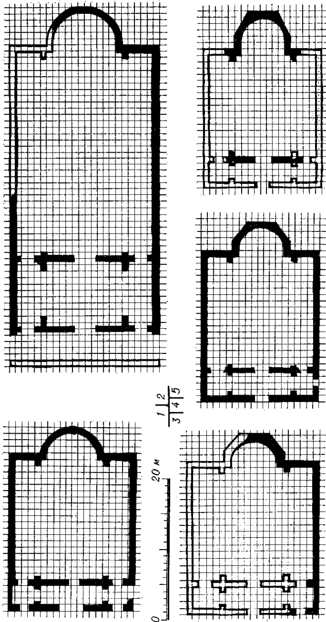
Рис. 3. Модульна побудова планів: 1 — «Базиліка в базиліці», 2 — «Уварівська базиліка», 3 — «Північна базиліка», 4 — «Базиліка 1932 р.», 5 — «Базиліка біля собору» (заливкою позначені існуючі залишки планів).
