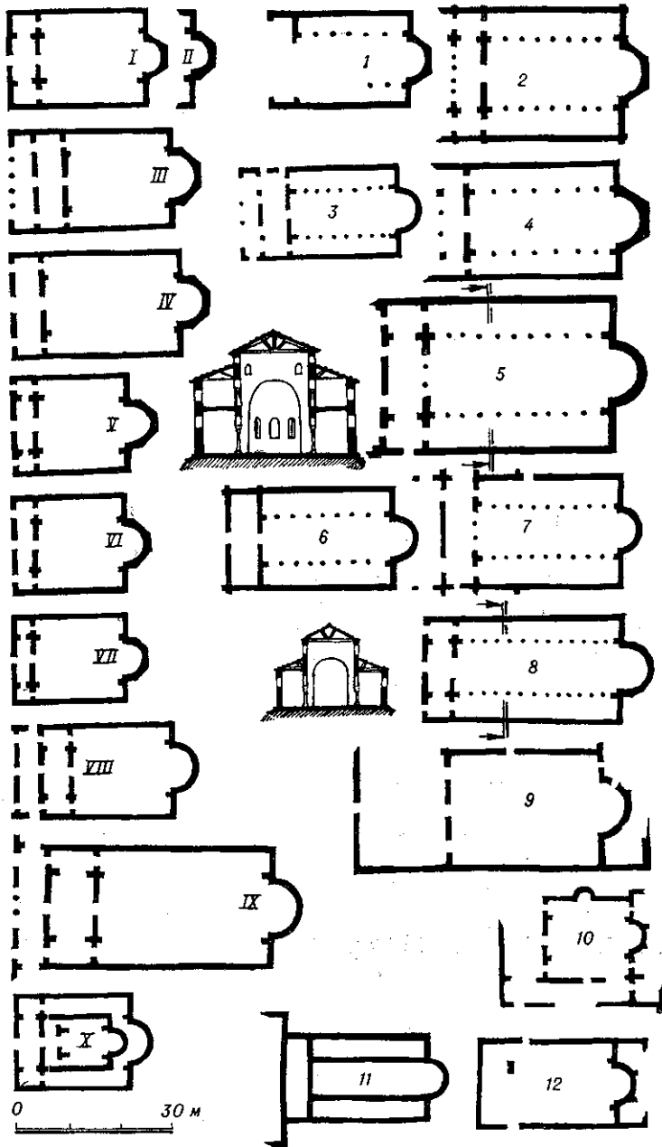
Рис. 1. Плани елліністичних базилік Криму (I—X) та їх аналогів в інших регіонах імперії (1—12); 1—базиліка на Мангуні, 11—«Базиліка на горбі», 111—«Східна базиліка», IV—«Західна базиліка», V—«Базиліка біля собору», VI—«Північна базиліка», VII—«Базиліка 1932 р.», VIII—«Базиліка 1935 р.», IX—«Уварівська базиліка», X—«Базиліка в базиліці». 1—Хісар, 4—базиліка св. Олени в Єрусалимі, 5—базиліка Ахіеропоетос у Салоніках, 6—базиліка на горбі Царевець в Турново, 7—базиліка «А» у Фтіотійських Фівах, 8—базиліка Аполлінарія Нового в Равенні, 9—базиліка в Корікосі, 10, 12—базиліки в Корасіоні, 11—базиліка в Пергамоні.
