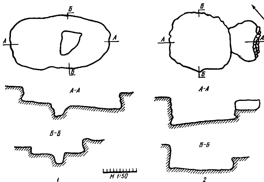
Рис. 2. Плани та розрізи скельних споруд (1, 2).
