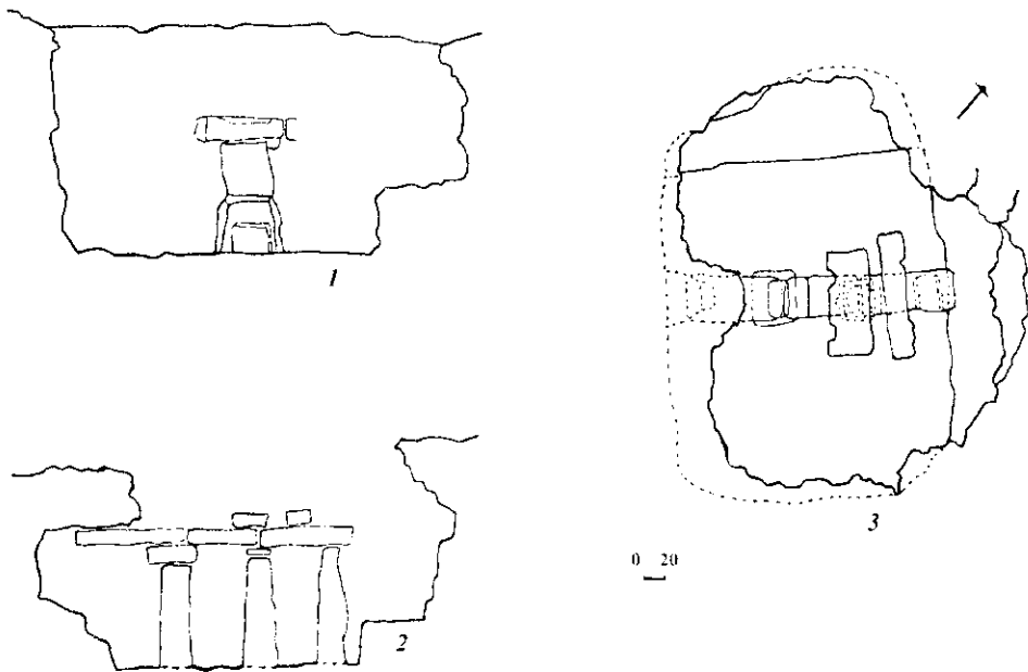
Рис. 1. Вхідний отвір (1), розріз (2) та план склепу.
