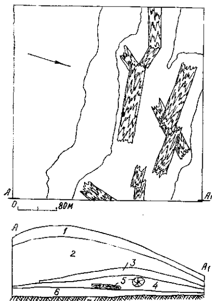
Рис. 3. «Мале» городище. Розріз валу та план обгорілих конструкцій: 1 — шар дерну; 2 — підзол; 3 — обгорілий шар; 4 — попіл; 5 — дерево; 6 — рівень стародавнього горизонту; 7 — материк.
