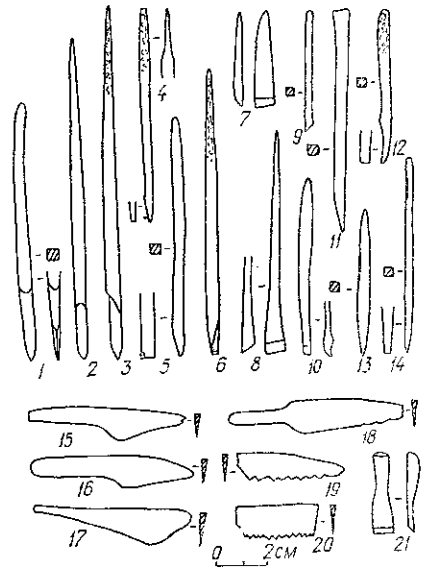
Рис. 2. Залізні знаряддя для різьблення, гравірування, пилиння кістки. 1—3 — скальпельоподібні різці; 4, 9, 11, 14 — прямі плоскі різці; 5, 10, 12 — різці для виїмочних робіт; 6 — кутовий різець; 7, 8 — косі різці; 13 — інструмент для гравірування; 15, 16, 17 — контурні ножі; 18 — підрізний ніж; 19, 20 — дрібнозубчасті пилки; 21 — косий різець з втулкою для рукоятки. 1, 19—21 — Люботинське городище; 2—18, 20 — Більське городище.
