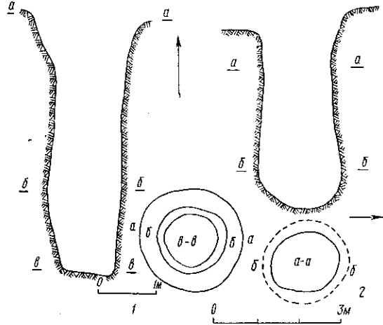
Рис. 21. Плани та розрізи цистерн: 1 — цистерна № 2; 2 — цистерна № 1.
