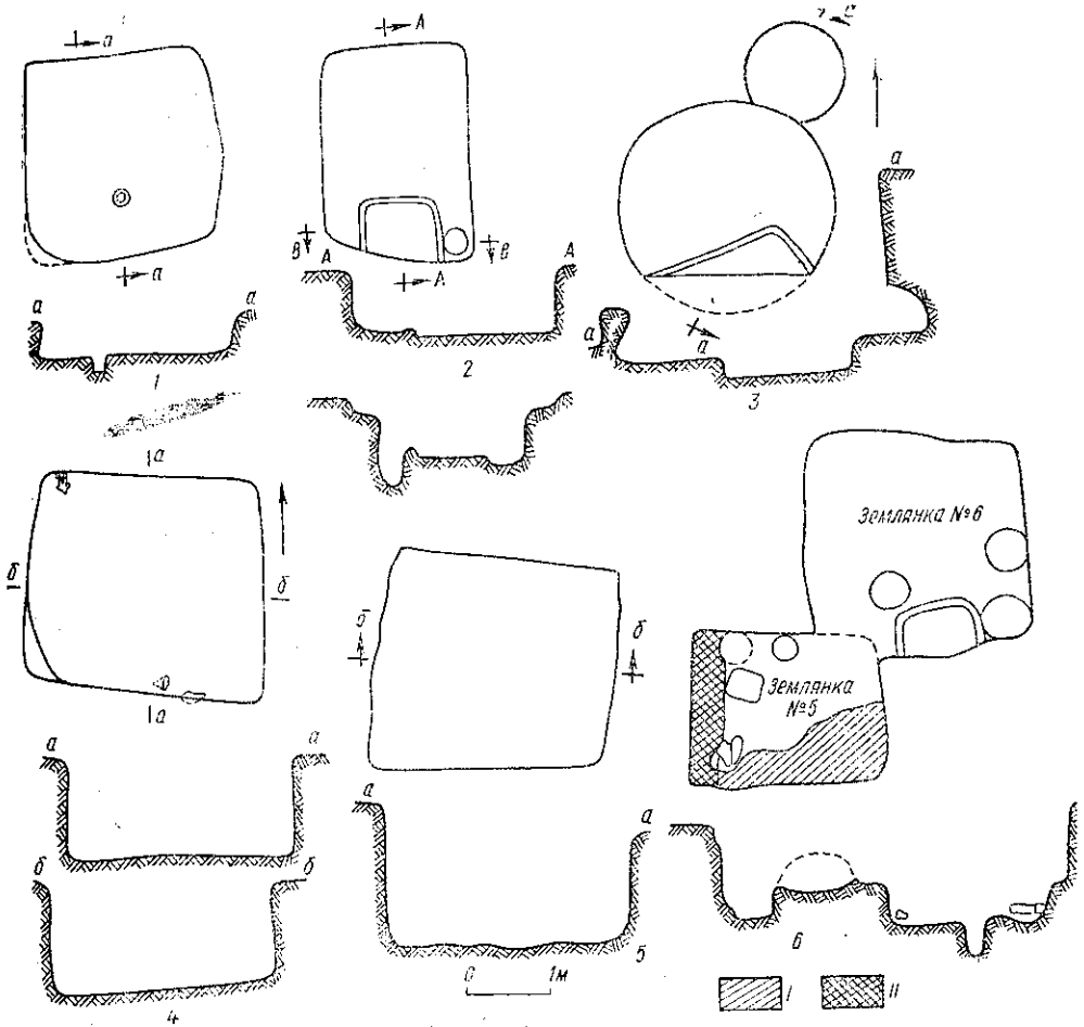
Рис. 5. Плани та розрізи земляних жител:
