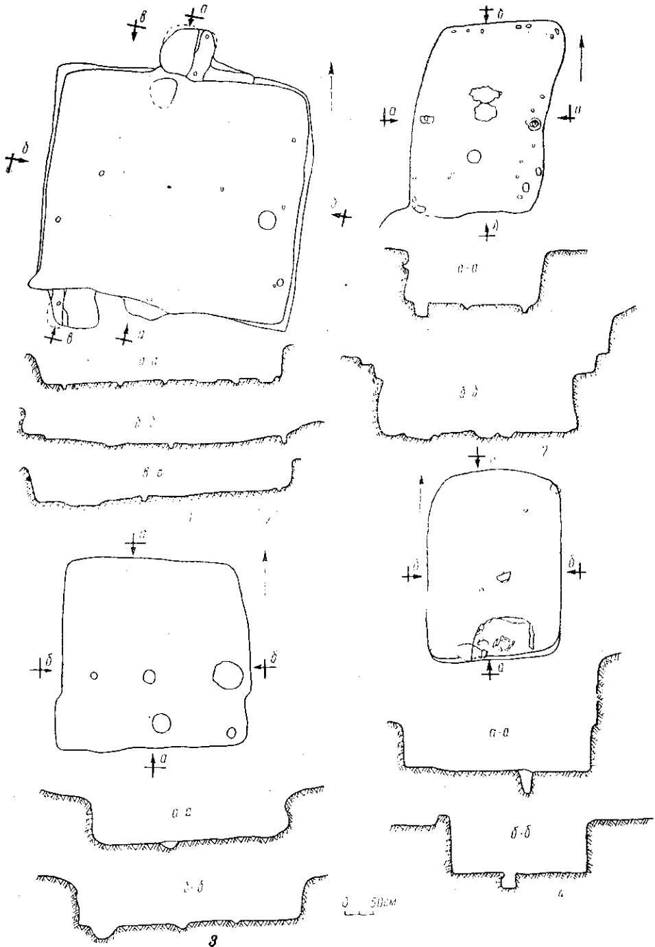
Рис. 6. Плани та розрізи земляних жител:
