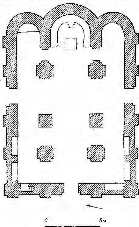
Рис. 24. Руїни шестистовпного храму XII ст. План.
