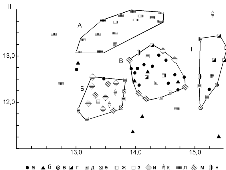
Рис. 2. Взаємостосунки антропологічних типів східних слов'ян доби Київської Русі за даними канонічного аналізу (за С. Г. Єфімовою, 1999)
