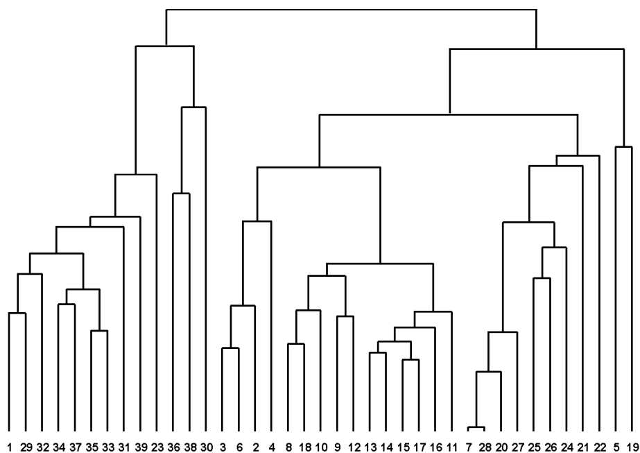
Рис. 5. Результати кластерного аналізу матриці відстаней Махаланобіса ( D^2 ) між середньовічними групами Європи (за С. Л. Санкіною і О. Г. Козінцевим, 1995)
