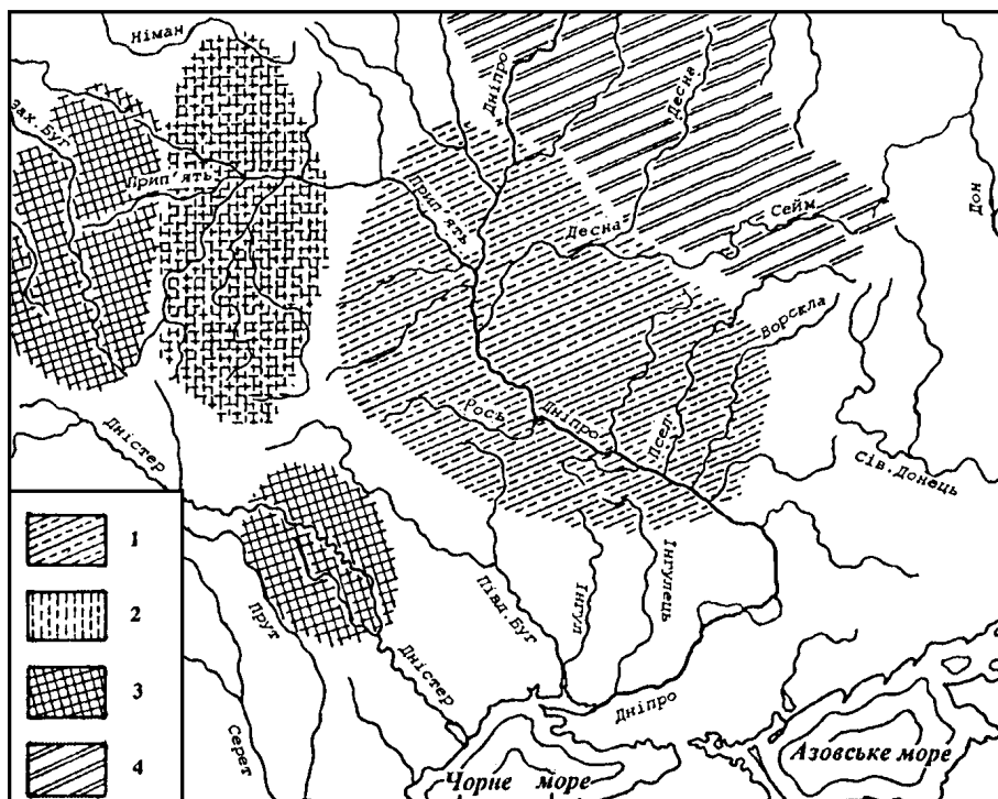
Рис. 1. Антропологічні типи давньоруського населення України (за Т. І. Алексєєвою, 1973) 1 — мезокефальний середньолиций; 2 — доліхокефальний широколиций; 3 — мезокефальний широколиций; 4 — доліхокефальний середньолиций
