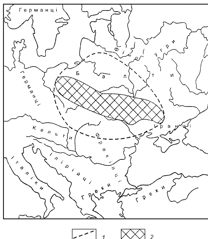
Рис. 3. Ймовірна «прабатьківщина» слов'ян (за Т. Алексеевою та В. Я. Алексеевим, 1989) 1 — за даними антропології; 2 — за даними археології
