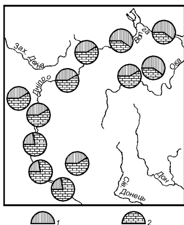
Рис. 4. Співвідношення основних морфологічних компонентів населення Східної Європи доби Київської Русі (за Т. І. Алексеевою, 1973) 1 — компонент з послабленим випинанням носа; 2 — компонент з сильним випинанням носа
