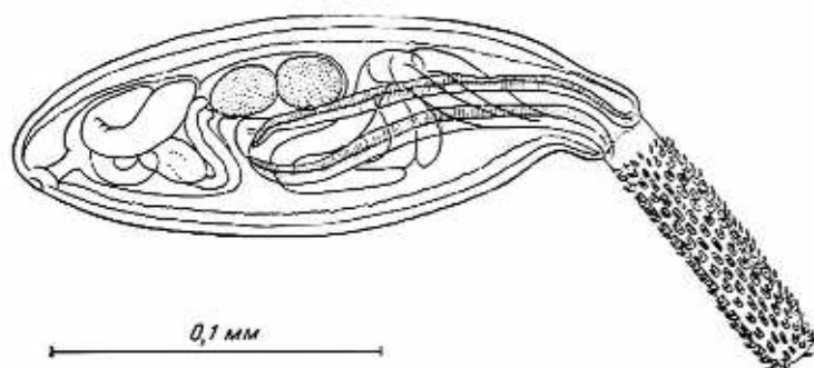
Рис. 2. Prosthynchus cylindraceus (Goetze, 1782). Цистакант.
