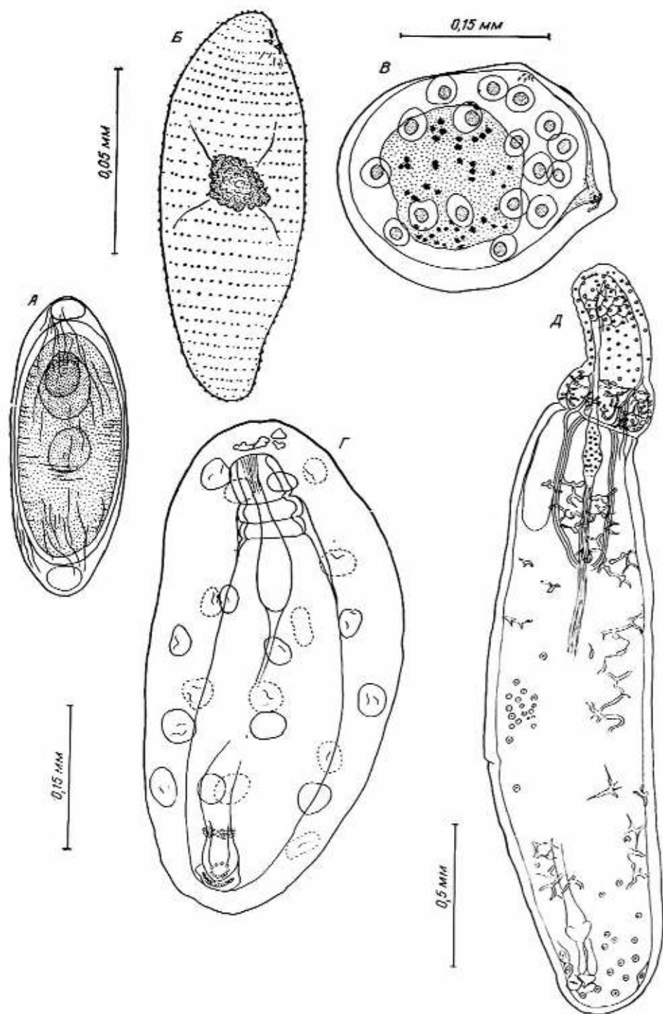
Рис. 1. Prosthorhynchus cylindraceus (Goetze, 1782). Стадии развития: а — яйцо; б — акантор; в — ранняя акантелла; г — средняя акантелла I; д — средняя акантелла II.
