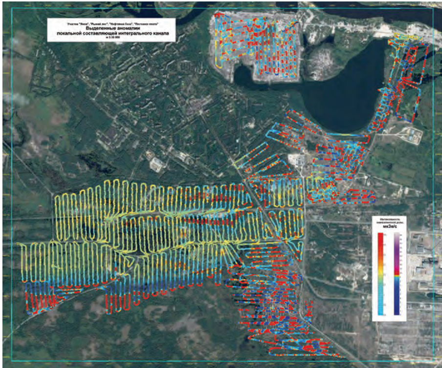
Рис. 4. Визначення радіаційних забруднень місцевості системою «Р-Навігатор»
