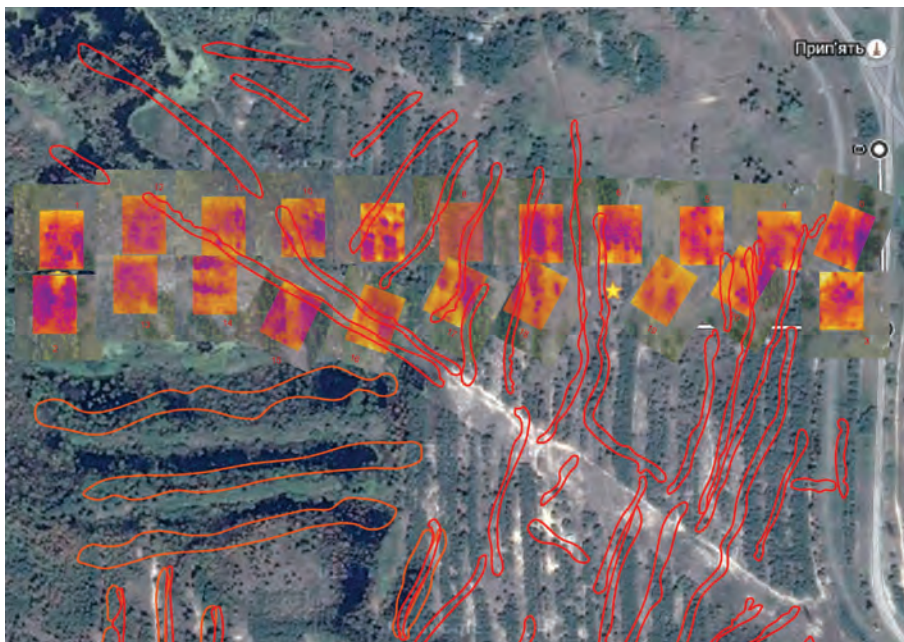
Рис. 5. Результати роботи тепловізійного каналу
