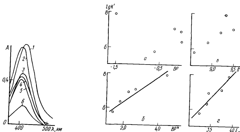
Рис. 1. Спектры поглощения комплексов К(ДВ18С6)БТС в хлороформе (1), в бензоле (2), в хлорбензоле (3), в четыреххлористом углероде (5), Na(ДВ18С6)БТС в толуоле (4) и Pb(ДВ18С6)(БКЗ) 2 в толуоле (6). C_M = 4 \cdot 10^{-3} М (6), 5 \cdot 10^{-3} (1), 1 \times 10^{-2} (2, 3), 5 \cdot 10^{-2} (5), 4 \cdot 10^{-1} (4); C_{БТС} = 4 \cdot 10^{-5} ; C_{БКЗ} = 5 \cdot 10^{-5} ; C_L = 1 \cdot 10^{-3} (1), 5 \cdot 10^{-4} (2, 4, 6), 5,9 \cdot 10^{-4} (3), 2,2 \cdot 10^{-4} М (5).
