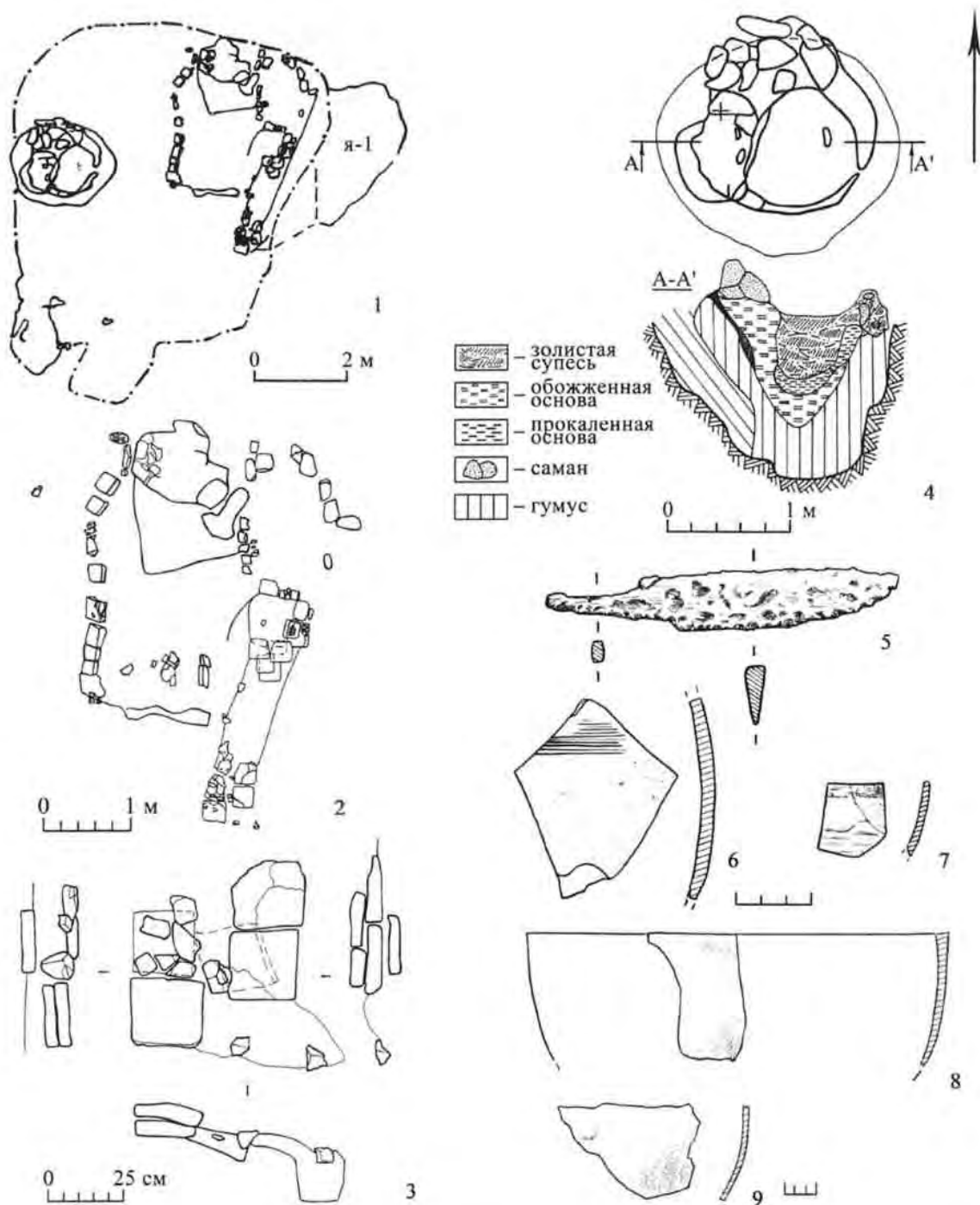
Рис. 4. Жилище 2: 1 – план помещения и конструкций; 2 – сооружение из кирпича (суфа) с очагом; 3 – южный край сооружения из кирпича, план и разрезы; 4 – тандыр, план и разрез; 5 – железный нож; 6 – фрагмент красноглиняного кувшина; 7 – фрагмент пиалы; 8, 9 – фрагменты чугунного котла
