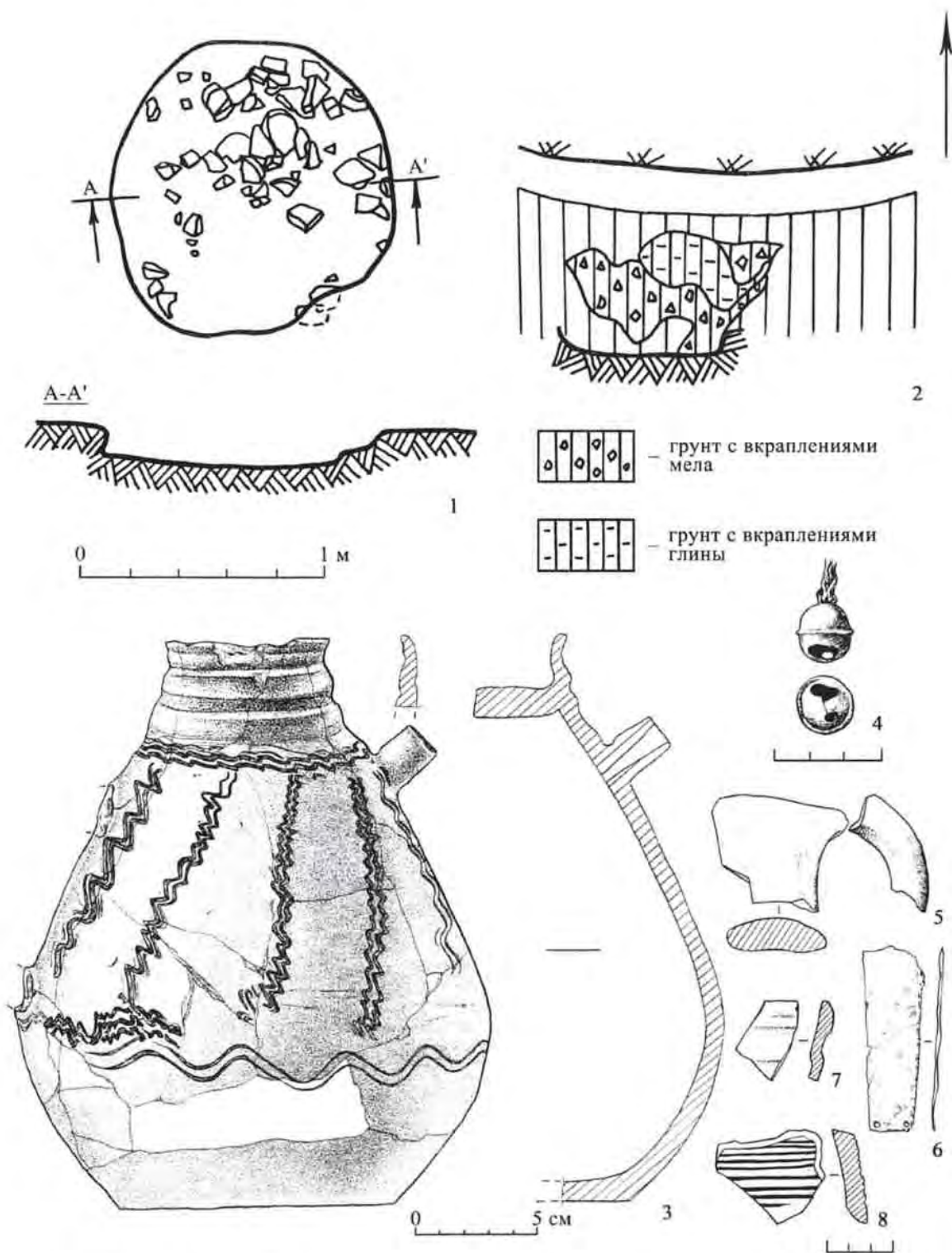
Рис. 9. Хозяйственная яма 4: 1 – план и разрез ямы; 2 – профиль заполнения ямы; 3 – кальян; 4 – бронзовый бубенчик; 5 – ручка от кувшина; 6 – железная пластина; 7, 8 – фрагменты керамики.
