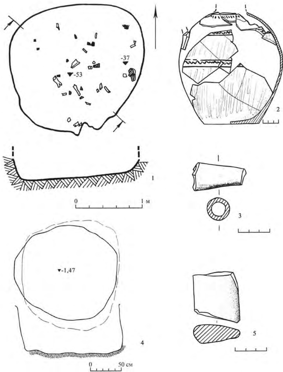
Рис. 8. Хозяйственная яма 3: 1 – план и разрез ямы; 2 – кумган; 3 – носик кумгана. Хозяйственная яма 5: 4 – план и разрез ямы; 5 – ручка сосуда золотоордынского времени.
