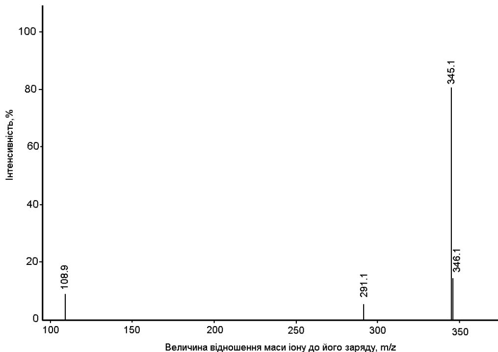
Рис. 2. Мас-спектр ГК 3 , що містить кластер молекулярного іона ( m/z = 345 ) та фрагментарні іони ( m/z = 291 , m/z = 109 ), одержаний під час хроматографічного розділення та ідентифікації суміші з плаваючих вай папороті Salvinia natans
