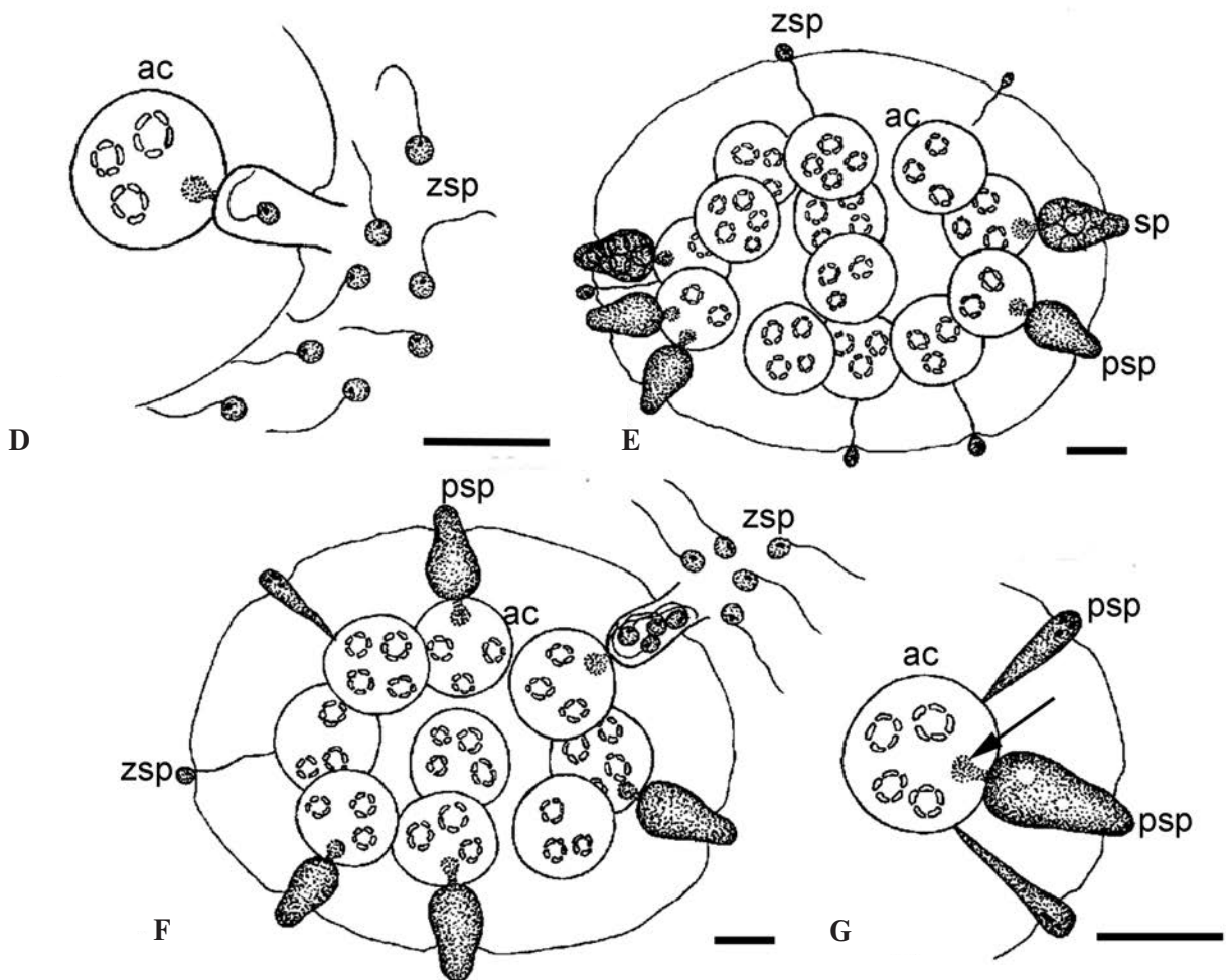
Рис. 3. Dangeardia mammilata на колонії Eudorina elegans . А, В: ураження клітини водорості (ac) зооспорами гриба (zsp) та утворення проспороангіїв (psp); С: зрілий зооспороангіій (sp) на ценобії (coe); Д: вихід зооспор (zsp); Е, F: загальний вигляд уражених ценобіїв; G: стадії формування спорангіїв (стрілкою позначено гаусторій). Масштаб: 10 мкм
