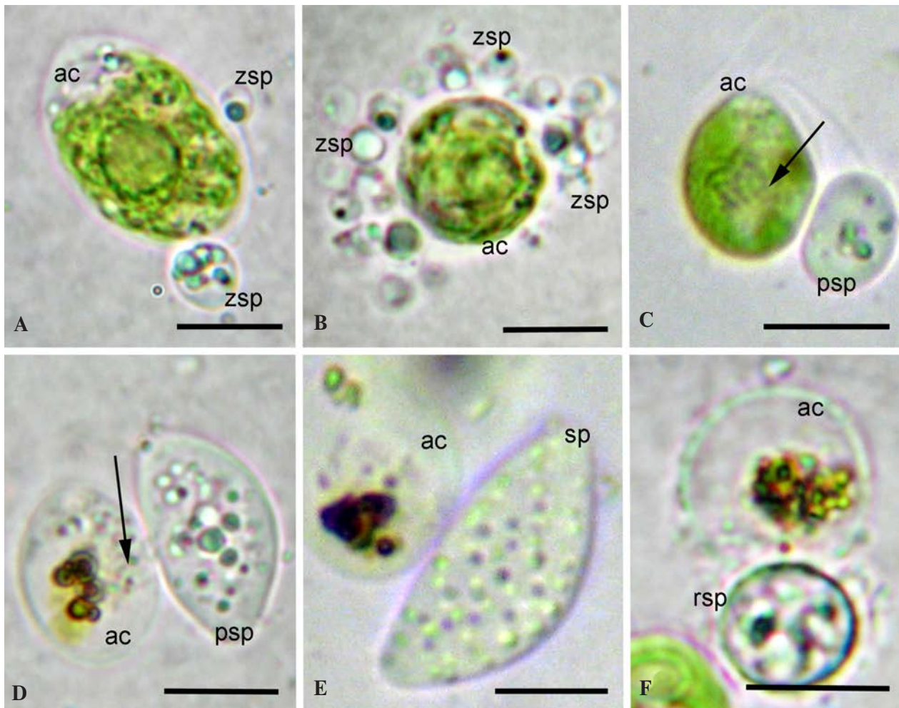
Рис. 5. Rhizophydium transversum на Chlamydomonas noctigama . А, В: ураження клітини водорості (ac) зооспорами гриба (zsp) (В – масове ураження); С, D: проспороангії (psp) на клітинах водорості (ac), стрілками позначено гаусторій (С) та "ризоди" (D); Е: зрілий зооспороангій (sp) на відмерлій клітині водорості (ac); F: клітина спокою (rsp) на відмерлій клітині водорості (ac). Масштаб: 5 мкм (А, В, D–F) та 10 мкм (С)
