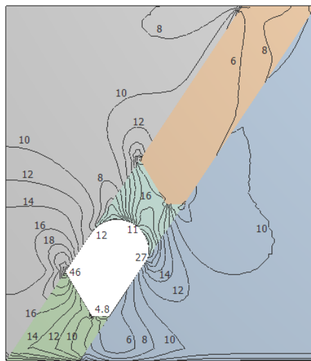
Рисунок 2 - Результати розрахунку і ізолінії головних напружень \sigma_1 гірського масиву при формуванні склепоподібної стелини: руда – 3P, порода в/б – 2П, порода л/б – 3П, тиск – P_1
