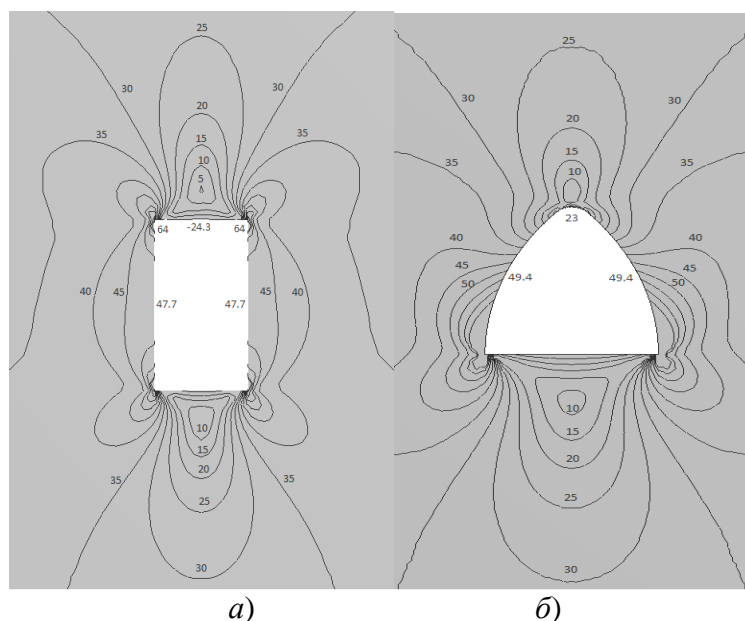
Рисунок 4 – Розподіл еквівалентних напружень навколо очисної камери: a – прямокутної форми; б – квазіпараболічної форми.
