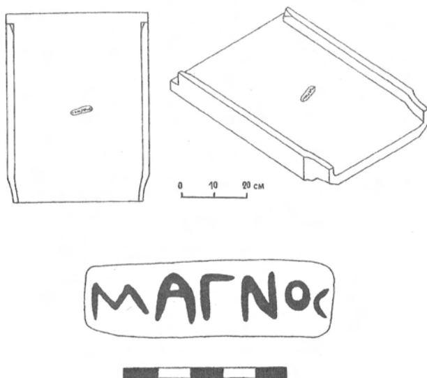
Рис. 1 Схема конструкции черепицы. Клеймо ΜΑΓΝΟΣ.
