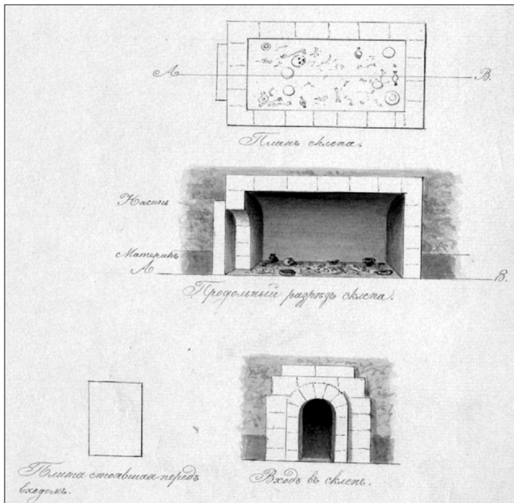
Рис. 8. Склеп VII в Артюховском кургане [Р. I, д. 568, л. 17 об.].
