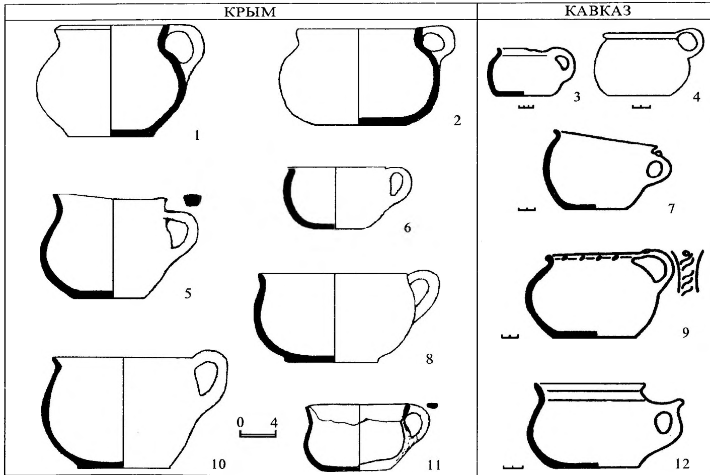
Табл. IX. Ковши типа 1.
