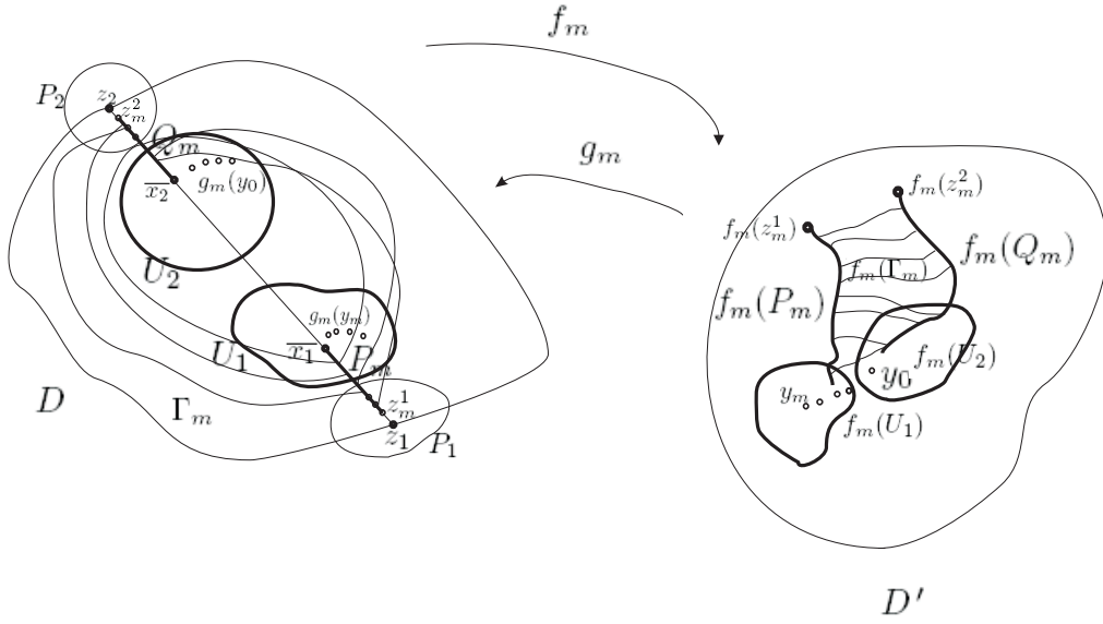
Рис. 1. К доказательству теоремы 1
