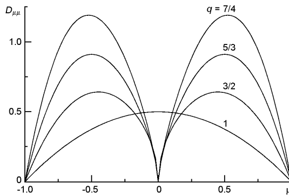
Рис. 4. Зависимость коэффициента диффузии КЛ D (44), (46) от косинуса питч-угла частицы для разных значений параметра q (числа у кривых)
