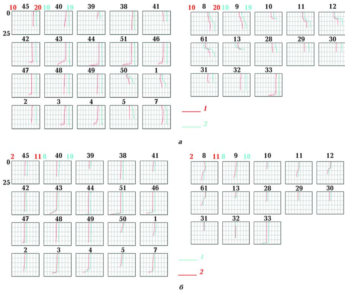
Рис. 4. Вертикальний розподіл: а — температури й солоності; б — розчиненого кисню і водневого показника. Полігон "Північний", 09—11.10.2018 р.
