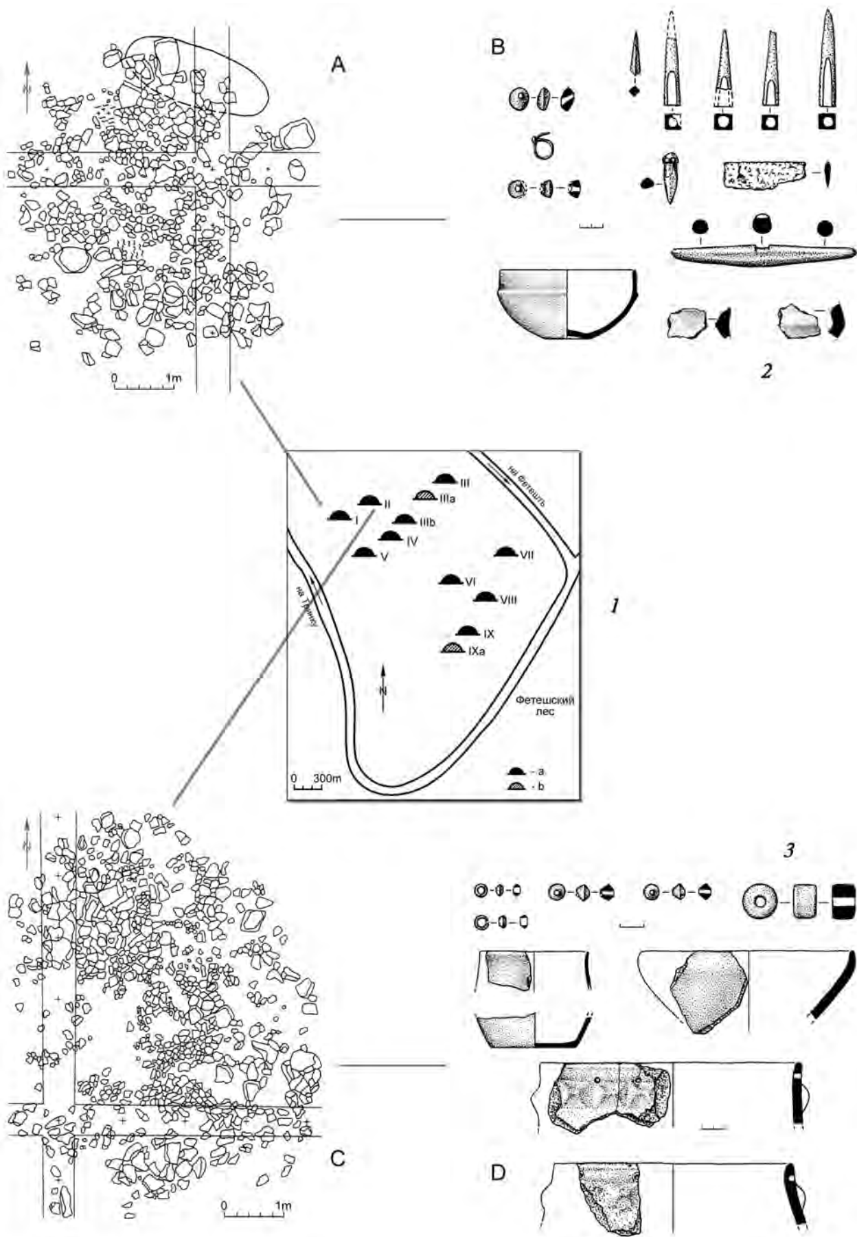
Рис. 2. Могильник Тринка-Друмул Фетештилоу. 1 – расположение курганов; 2 – курган I (план и инвентарь); 3 – курган II (план и инвентарь).
