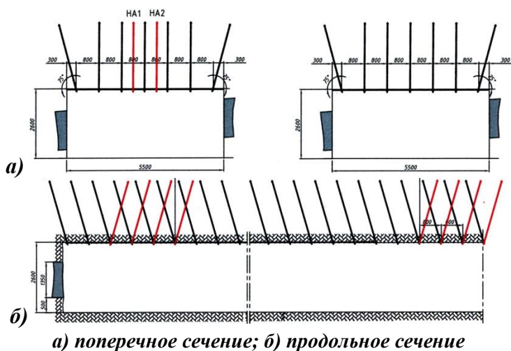
Рисунок 2. Схема установки АК
