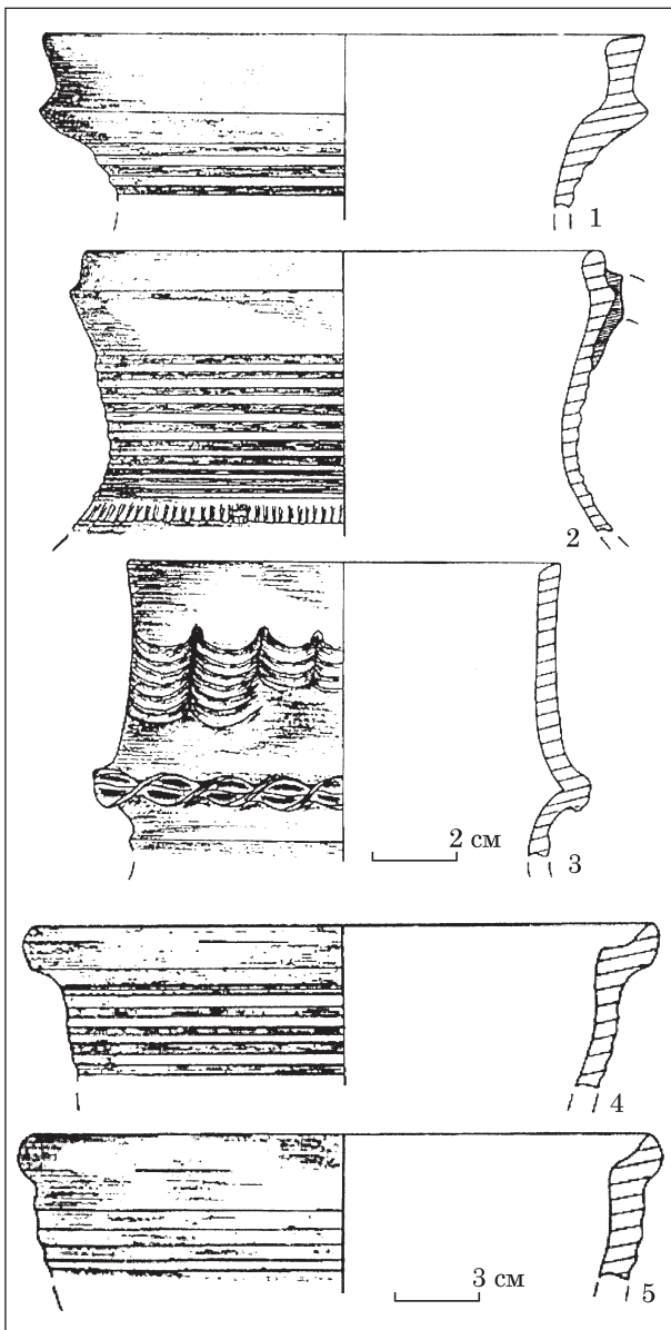
Рис. 13. Глеки підтипу I.2, типів II—III та ринки
