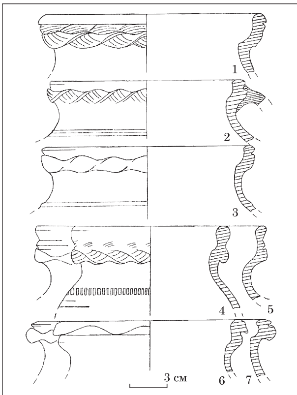
Рис. 9. Горщики підтипу V.1
