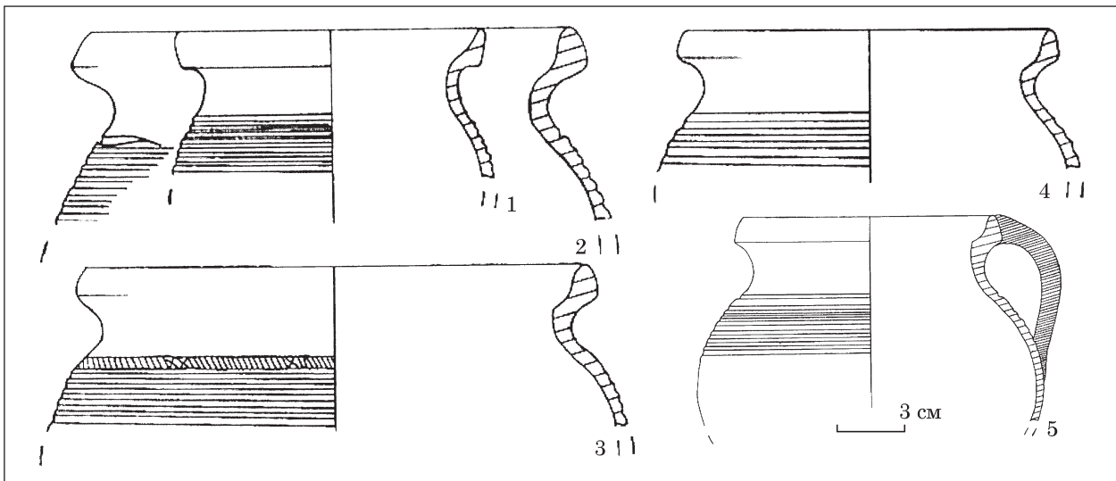
Рис. 4. Горщики типу III
