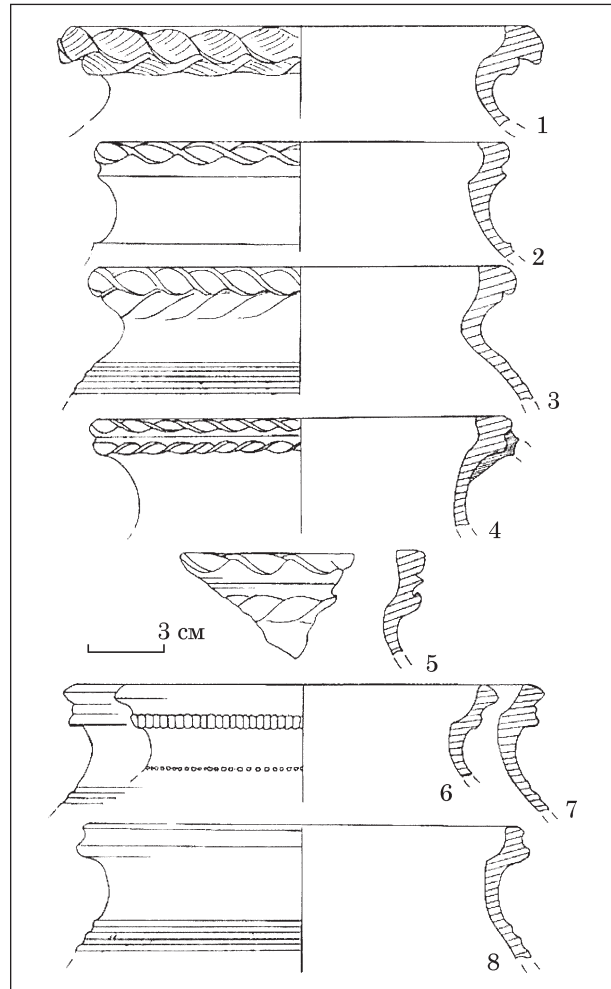
Рис. 10. Горщики підтипів V.2 та V.3
