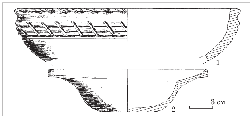
Рис. 14. Миска і тарілка
