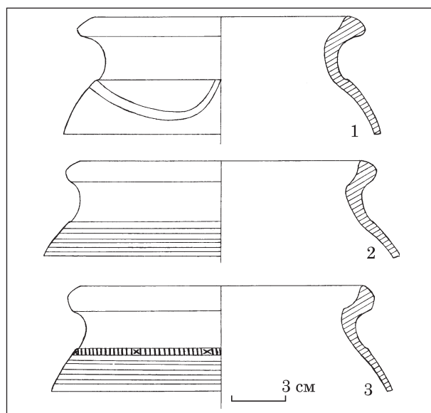
Рис. 6. Горщики підтипу IV.2
