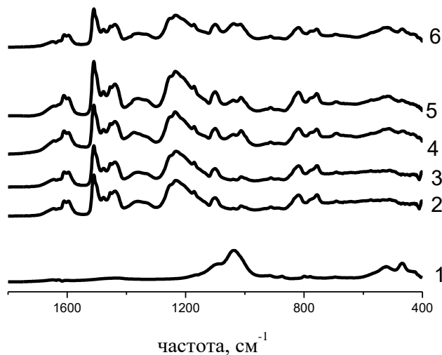
Рис. 1. Вплив кількості введеного монтмориллоніта на структуру олігофенілена, де 1 – спектр монтмориллоніта, 2 – спектр фенілену, 3, 4, 5, 6 – спектр олігомера, що містить 5, 10, 20, 30 гр монтмориллоніта відповідно
