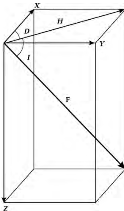
Рис. 1. Разложение вектора напряженности геомагнитного поля на составляющие.
