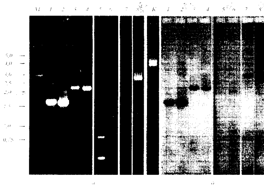
Рис. 4. Гель-электрофорез Southern-гипризации по Сухареву с кДНК IGF-1 клонированной продукции амплификации фрагментов генов IGF-1 различных рыб. Нечетные дорожки — первый этап амплификации, четные — второй этап. Дорожки 1 и 2 — окунь, 3 и 4 — судак, 5 и 6 — щука, 7 и 8 — плотва; К — контрольная реакция первого этапа на ДНК из мозга кельт; М — стандарт молекулярной массы, размер фрагментов ДНК в п.е. и в указан слева.
