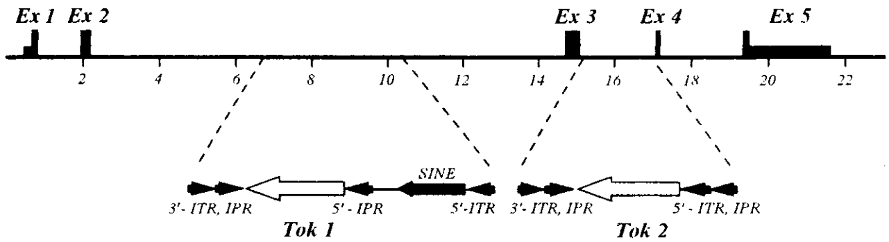
Рис. 1. Схема гена инсулиноподобного фактора роста 1 кеты. Экзоны (Ex1—Ex5) обозначены черными прямоугольниками, интроны — тонкой линией. Масштаб (тыс. п. н.) приведен под схемой гена. Гены транспозазы транспозонов Tok1 и Tok2 обозначены крупными белыми стрелками, ретротранспозонподобный элемент SINE — темной стрелкой. Инвертированные внешние (ITR) и внутренние (IPR) повторы транспозонов обозначены черными стрелками
