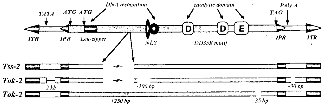
Рис. 2. Общая схема Tc1-подобного транспозона позвоночных [8] и схема транспозонов SALT(Tss2), Tok1 и Tok2. ITR — инвертированный внешний повтор; IPR — инвертированный внутренний повтор. Указан размер наиболее крупных вставок/делений
