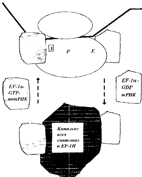
Рис. 3. Цикл комплекса EF-1\alpha — тРНК. тРНК в E сайте рибосомы взаимодействует с EF-1\alpha — GDP. Неканонический тройной комплекс теряет средство к рибосоме и взаимодействует с макромолекулярным агрегатом, содержащим стабильный мультисинтезазный комплекс, свободные аминоксил-тРНК синтетазы и EF-1\alpha бд. Внутри мультисинтезазного ассоциата происходит синтез аминоксил-тРНК и GTP/GDP-обмен в EF-1\alpha . Образовавшийся канонический тройной комплекс уходит из комплекса и взаимодействует с A сайтом рибосомы
