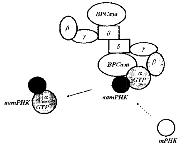
Рис. 2. Ченелинг тРНК в комплексе валил-тРНК синтетазы (VPSазы) с EF-1αβγδ . тРНК Val взаимодействует с валил-тРНК синтетазой, находящейся в комплексе с EF-1αβγδ . Одновременно происходят ферментативный синтез валил-тРНК и GTP/GDP-обмен в молекуле EF-1α . Взаиморасположение валил-тРНК синтетазы и EF-1α в комплексе таково, что образовавшаяся валил-тРНК сразу же формирует комплекс с EF-1α — GTP. Этот комплекс диссоциирует в раствор и направляется к А сайту рибосомы
