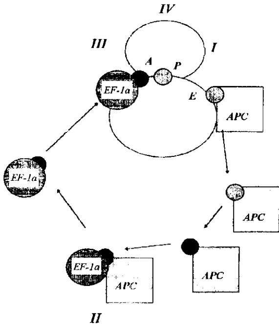
Рис. 1. Ченелинг тРНК в цикле трансляции. Деацилированная тРНК, находящаяся в Е сайте рибосомы (I), не диссоциирует в раствор до взаимодействия с аминоксил-тРНК синтетазой (APC). Происходит синтез аминоксил-тРНК, и аминоксил-тРНК передается на EF-1α — ГТР (II). Образовавшийся комплекс EF-1α — ГТР — аминоксил-тРНК взаимодействует с А сайтом рибосомы (III). Внутририбосомный путь тРНК от А до Е сайта происходит по классической схеме (IV)
