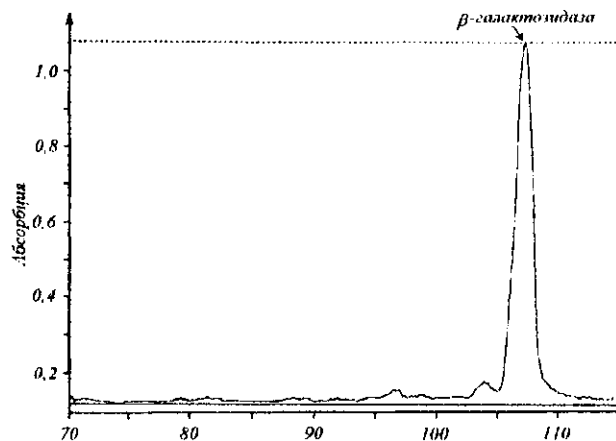
Рис. 2. Денситограмма с электрофорезом препарата \beta -галактозидазы после очистки лиганд-аффинной хроматографией. Содержание \beta -галактозидазы в препарате составляет 98 % от общего белка
