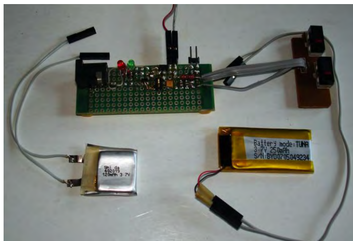
РИС. 5. Експериментальний макет вузла живлення сенсора
