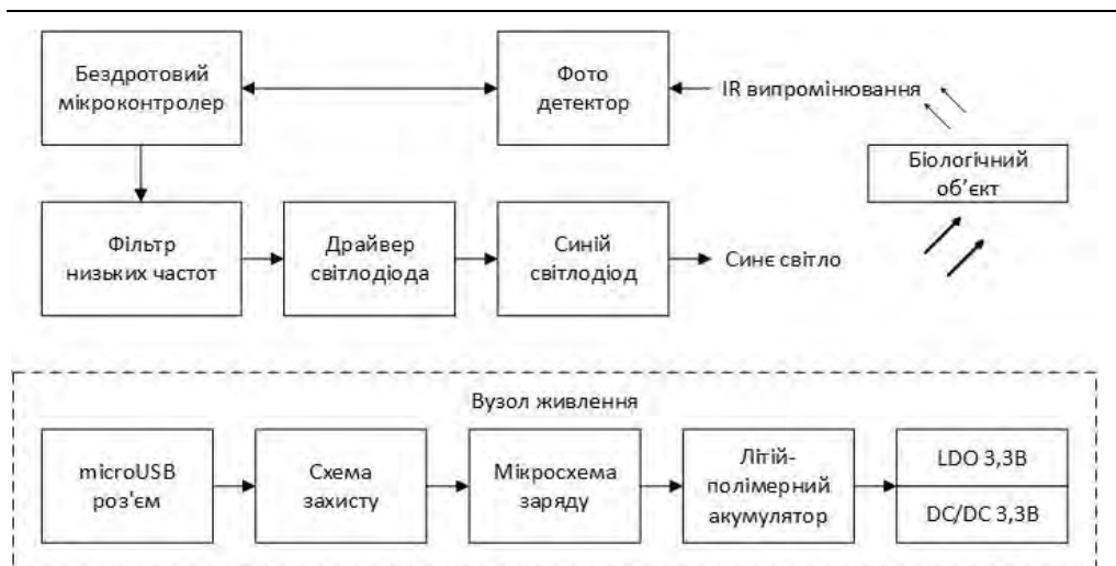
РИС. 1. Структурна схема бездротового інтелектуального сенсора
